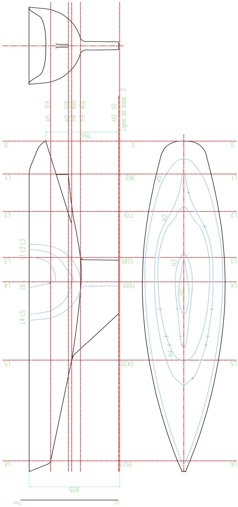
Demi largeur extérieur coque jauge
